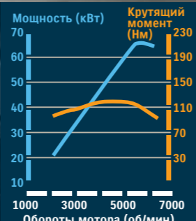
1,2-литровый бензиновый двигатель
