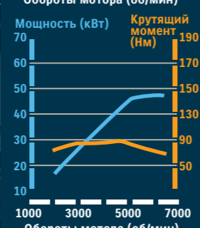
1,0-литровый бензиновый двигатель
